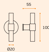
IN.00.173 STOUT Material: EN 1.4301 - Satinado / Satin / Satin Fixo / Fixed / Fijo
