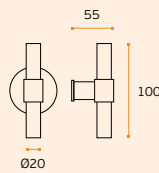
IN.00.172 STOUT Material: EN 1.4301 - Satinado / Satin / Satin RB08M - Roseta standard / Standard rose
