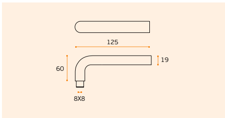
IN.00.028 Material: EN 1.4301 Satinado / Satin / Satin RB08M - Roseta standard / Standard rose
