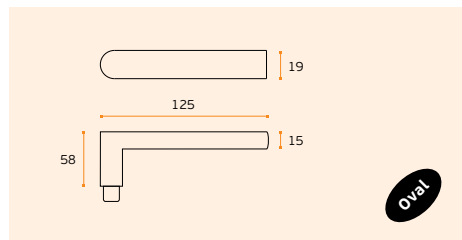
IN.00.031 Material: EN 1.4301 - Satinado / Satin / Satin RB08M - Roseta standard / Standard rose
