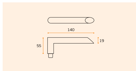
IN.00.035 Material: EN 1.4301 - Satinado / Satin / Satin RB08M - Roseta standard / Standard rose
