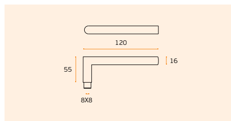
IN.00.036 Material: EN 1.4301 Satinado / Satin / Satin RB08M - Roseta standard / Standard rose
