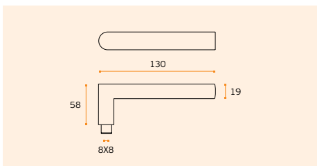
IN.00.030 Material: EN 1.4301 - Satinado / Satin / Satin RB08M - Roseta standard / Standard rose
