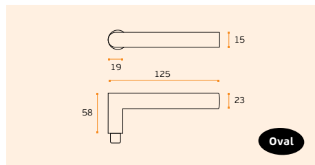
IN.00.032 Material: EN 1.4301 Satinado / Satin / Satin RB08M - Roseta standard / Standard rose
